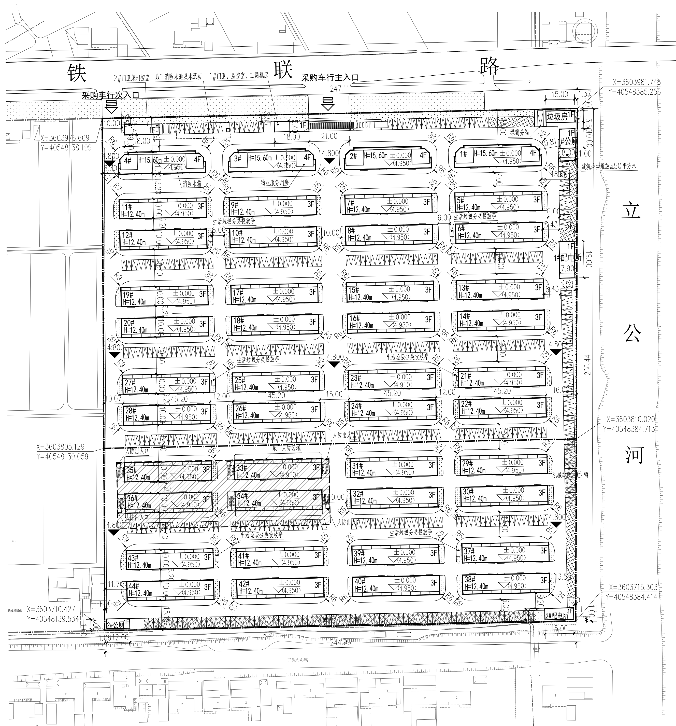
总平面图 1:1000
