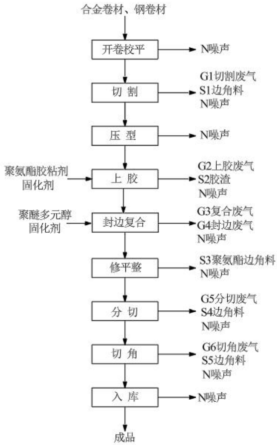
图 2-1 金属饰面复合板生产工艺流程图
