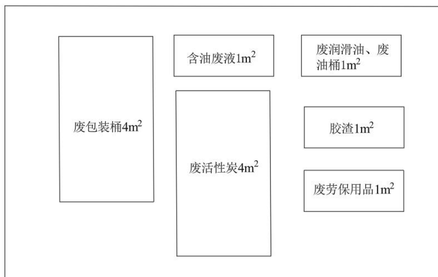
图 4-6 危废仓库布置图
