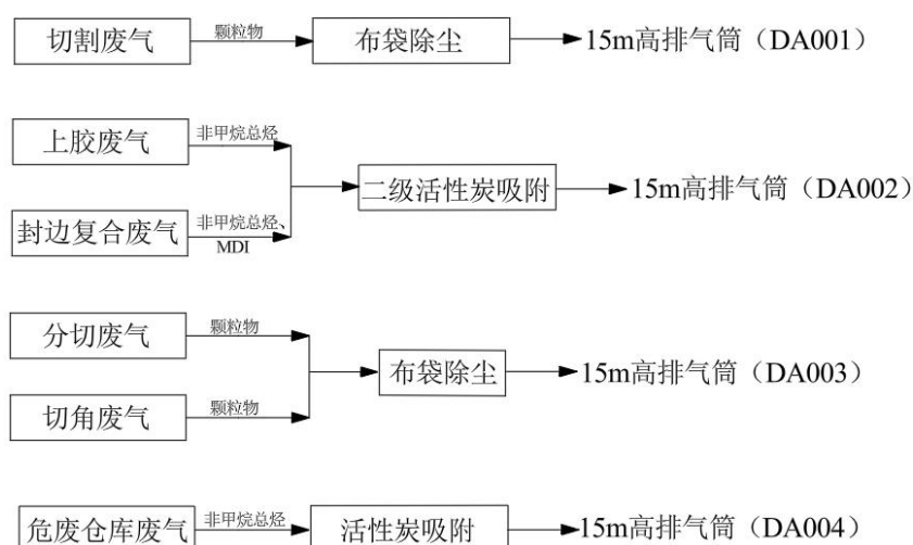
图 4-1 本项目废气收集、处理方式示意图
