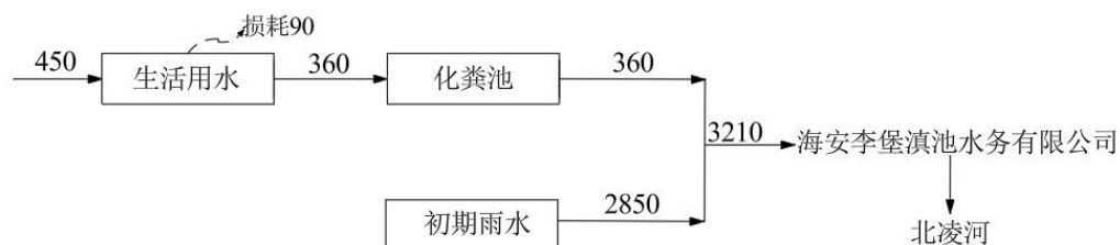
图 2-2 本项目营运期水平衡图 (单位: t/a)
