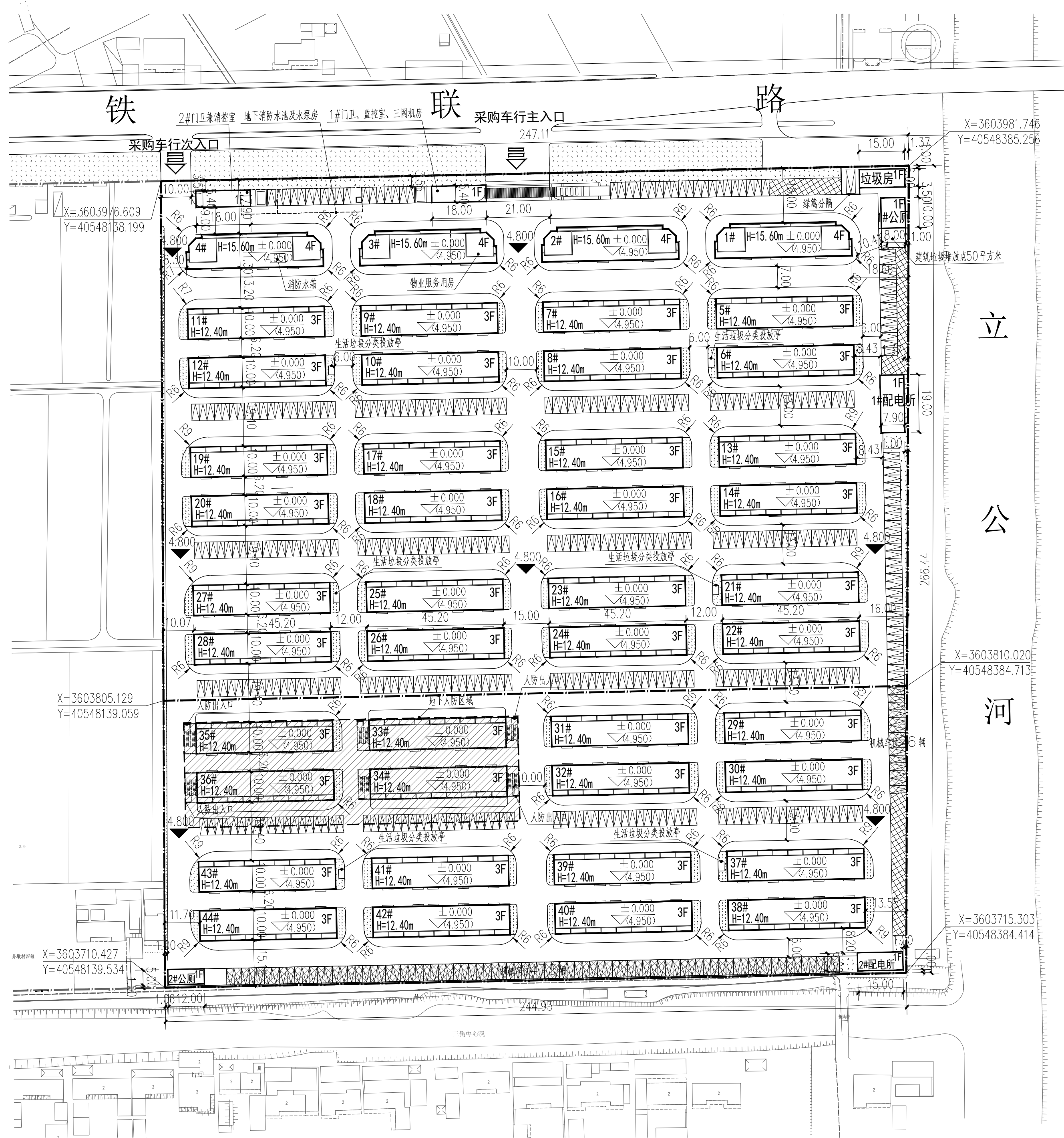
总平面图 1:1000
