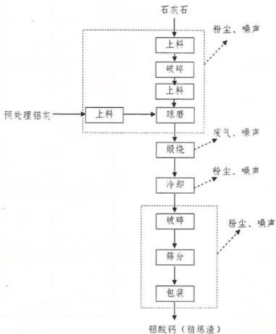
铝酸钙生产系统工艺及产排污环节图
