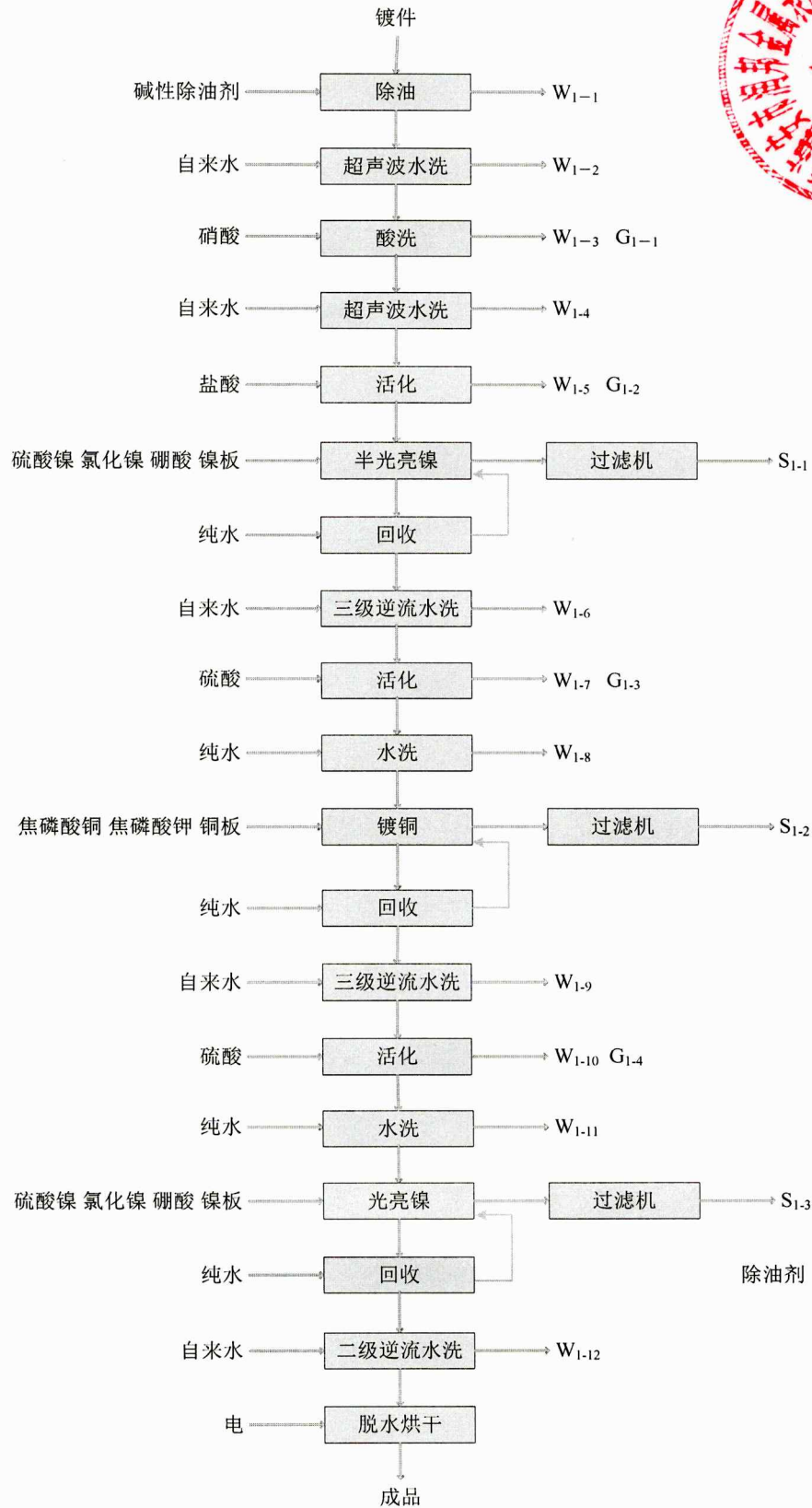
镍铜镍电镀生产线生产工艺流程图
