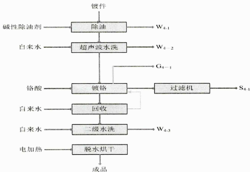
电镀铬生产线生产工艺流程图
