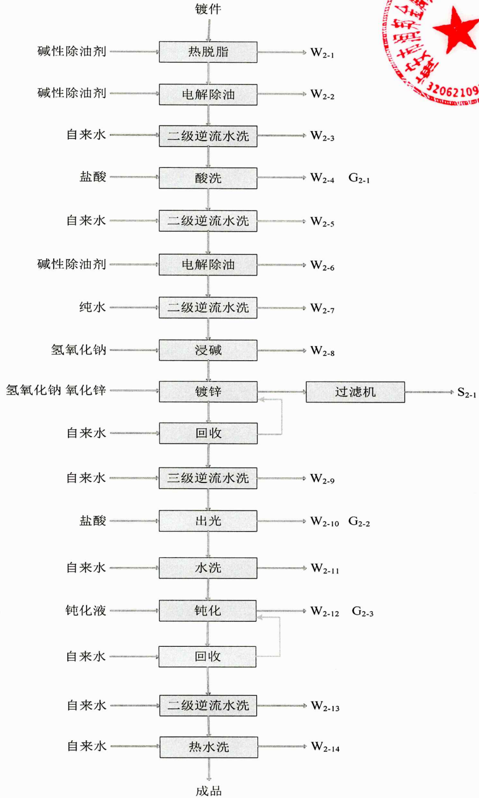
电镀锌生产线生产工艺流程图
